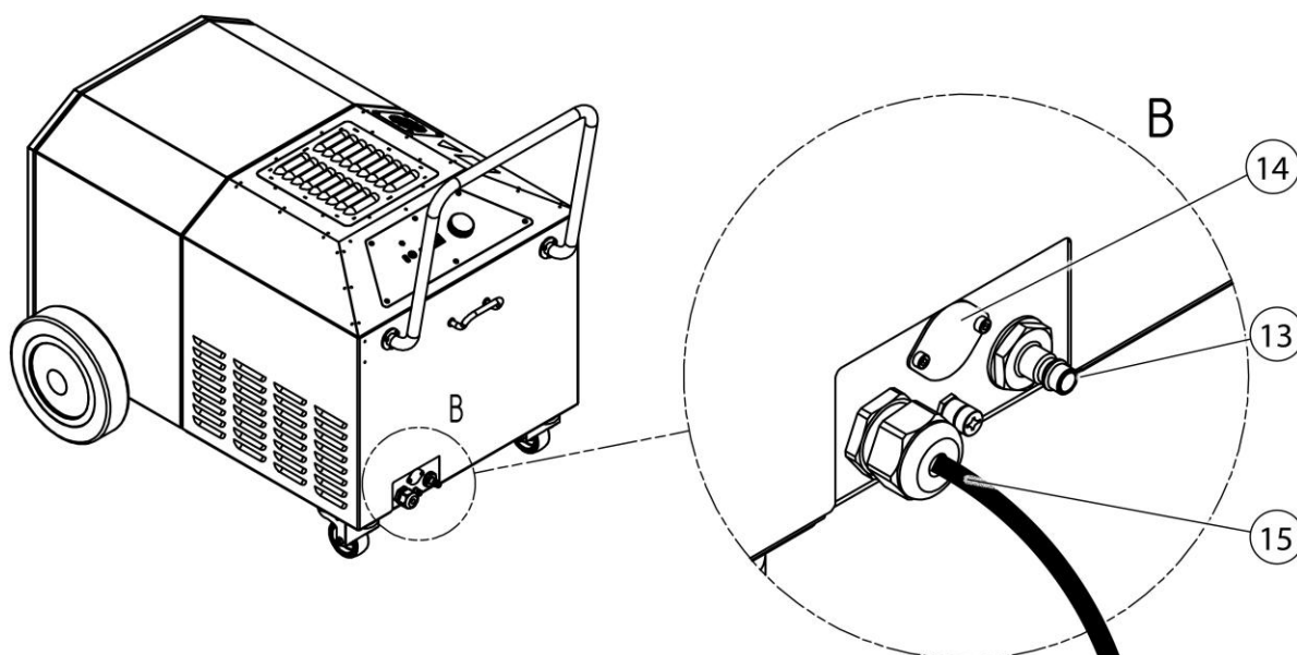
Afb. 2: Aansluitingen
