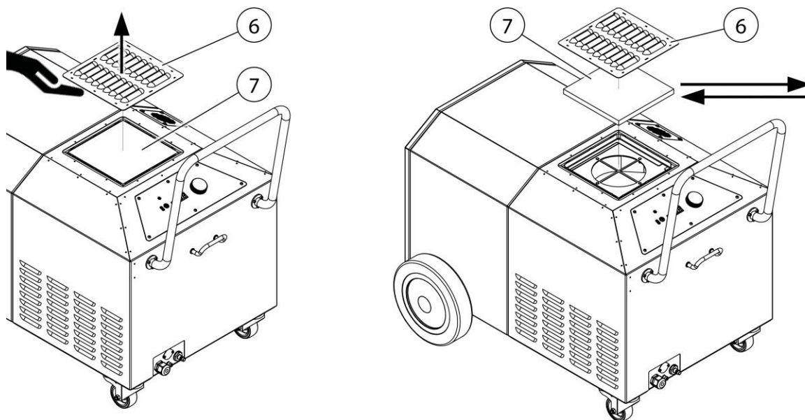
Afb. 8: Filtermat van de motorkoeling vervangen
