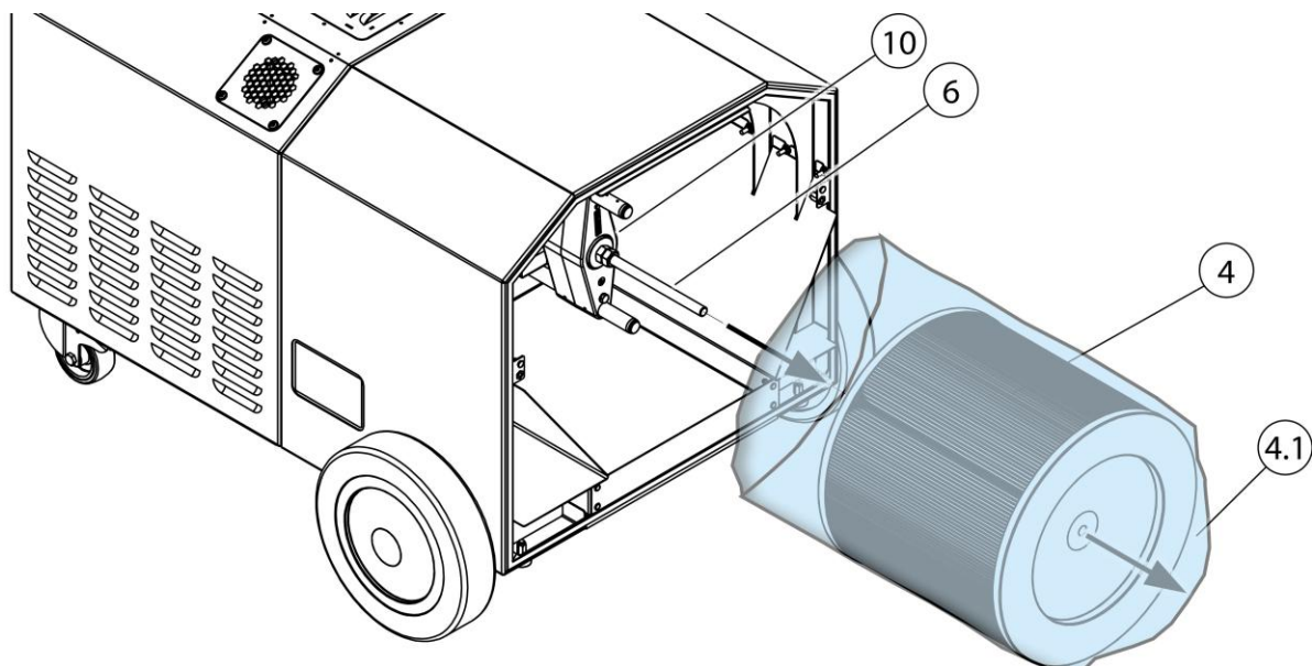
Afb. 11: Hoofdfilter verwijderen
