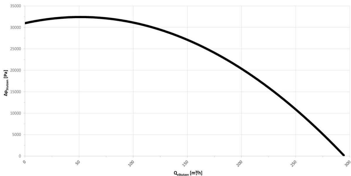
Afb. 16: Karakteristiek
